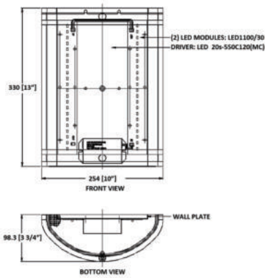
WS-T7572LED02 Dimension mm | 254(W) x 330(L) x 98(D) inch | 10"(W) x 13"(L) x 3.8"(D)
