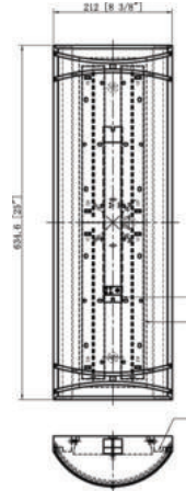
WS-705072LED04 Dimension mm | 212(W) x 92.5(D) x 635(L) inch | 8.35"(W) x 3.6"(D) x 25"(L)
