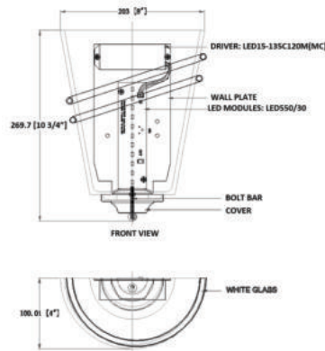
WS-T9806-LED01 Dimension mm | 203(W) x 270(L) x 100(D) inch | 8"(W) x 10.8"(L) x 4"(D)
