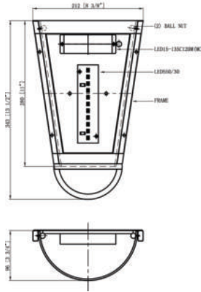
WS-T10412ALE01 Dimension mm | 212(W) x 343(L) x 104(D) inch | 8.35"(W) x 13.5"(L) x 4.1"(D)
