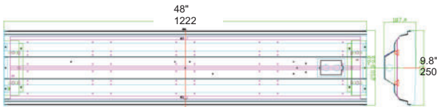
SHB4-16LED16 / SHB4-80LED08 Dimension mm | 1222(L) x 250(W) x 107(D) inch | 48"(L) x 9.8"(W) x 4.2"(D)
